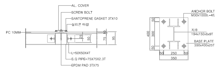
BASE PL. 상세
