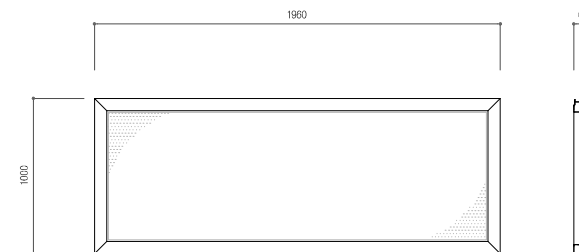
투명형 방음판 상세
